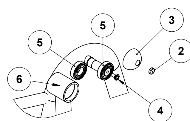
DETALHE D ESCALA 2 : 15
